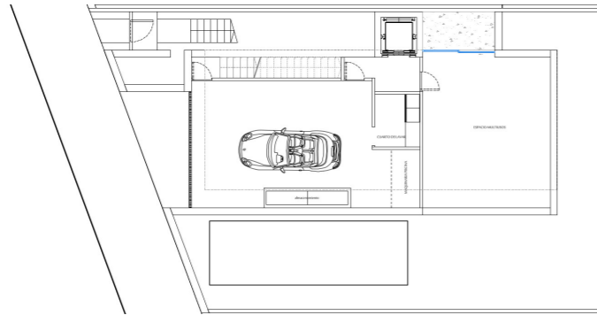
Planta sótano
