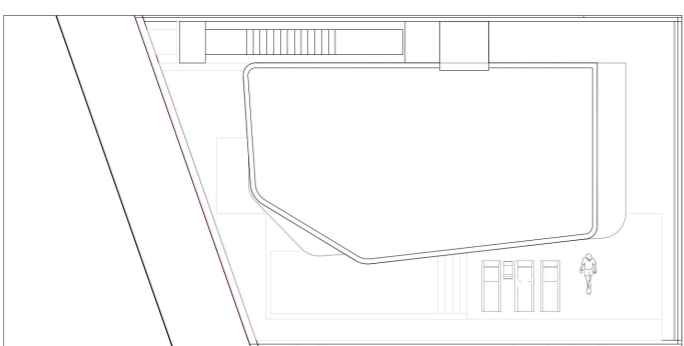
Planta cubierta
