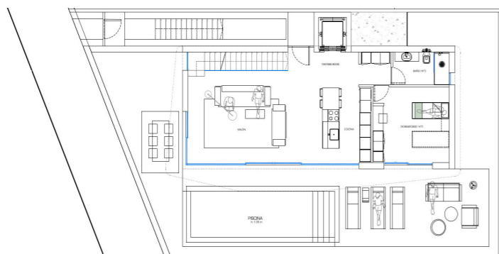
Planta baja
