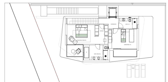
Planta alta
