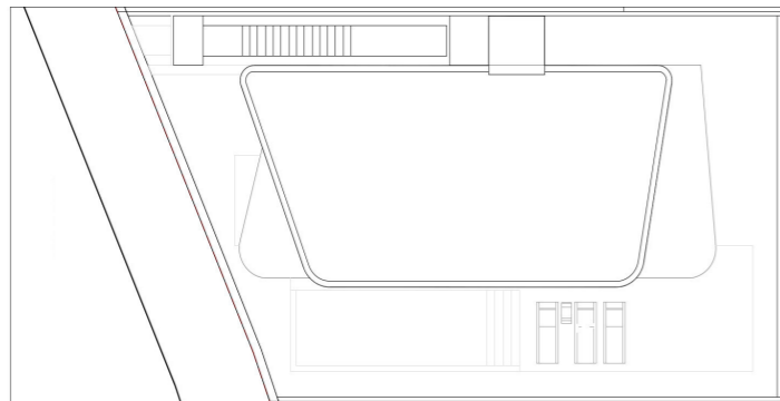
Planta cubierta
