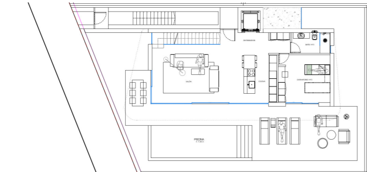
Planta baja
