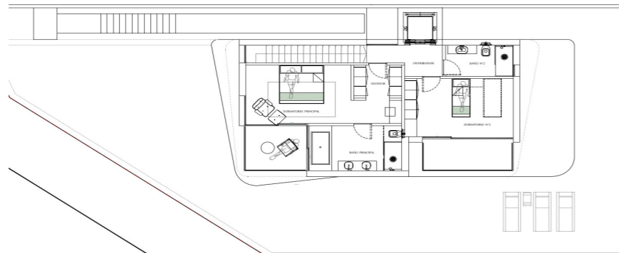
Planta alta
