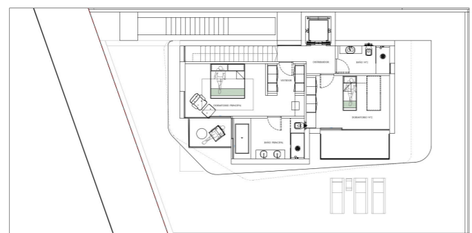
Planta alta
