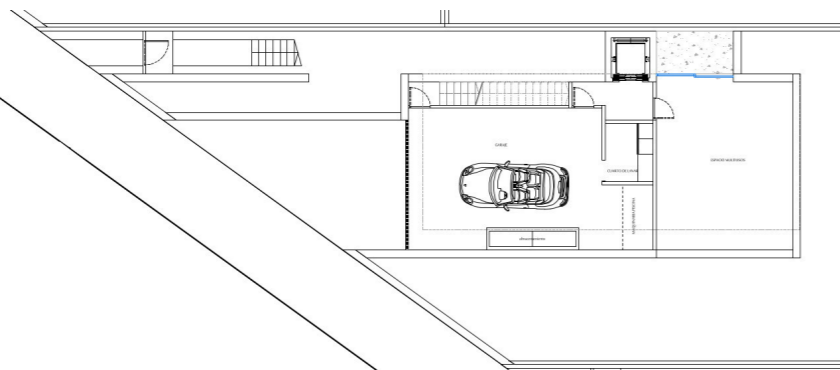
Planta sótano
