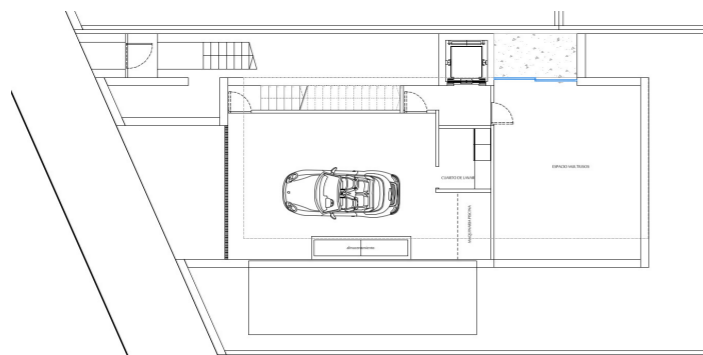
Planta sótano
